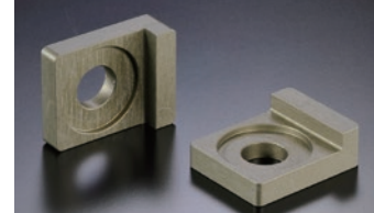
[38025] チェーン引きコマ T/S STD JAN.4522285380258 ¥2,400 (税抜) A2017材 ハードアルマイト仕上げ (汎用)
