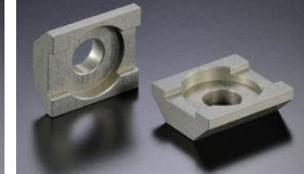
[38026] チェーン引きコマ T/S OW JAN.4522285380265 ¥3,600 (税抜) A2017材 ハードアルマイト仕上げ (汎用)
