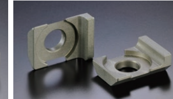
[38029] チェーン引きコマ T/Sミニ OW JAN.4522285380296 ¥3,600 (税抜) A2017材 ハードアルマイト仕上げ (汎用)
