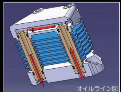
オイルライン図
