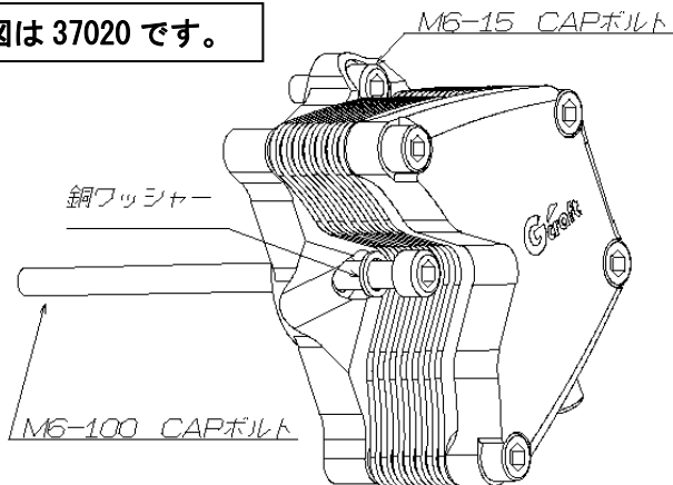
フィン数 11
